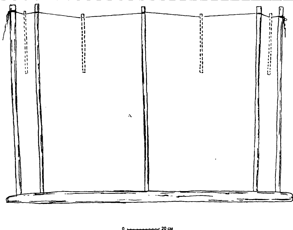
Илл. 11. Вероятная реконструкция предмета из-под днища колоды (№ 11—13).
